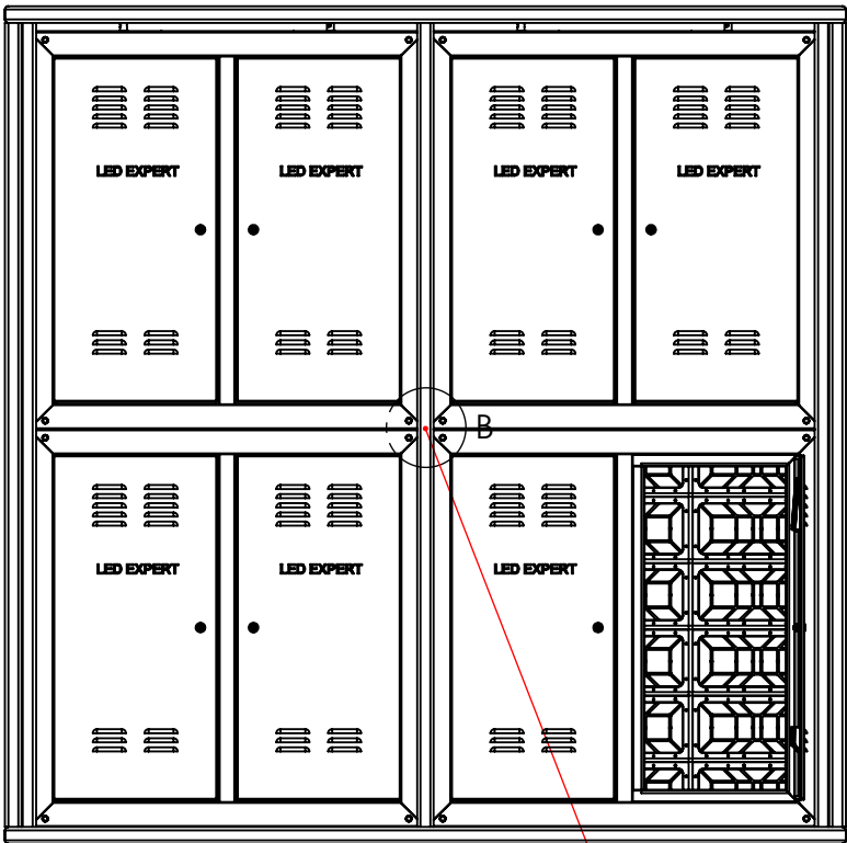
Vista traseira
